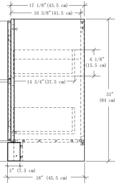
Side View / Vue de côté
