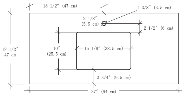
Vanity Top / Dessus du meuble-lavabo
