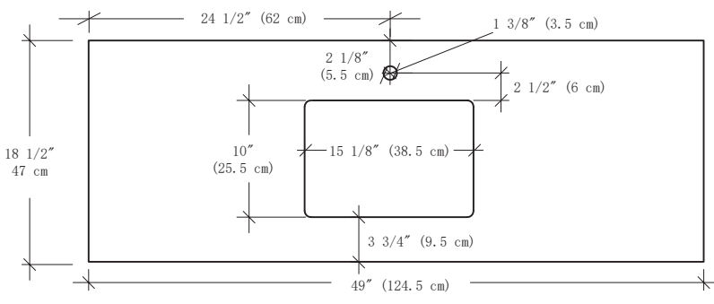
Vanity Top / Dessus du meuble-lavabo
