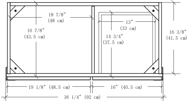
Front View / Vue avant
