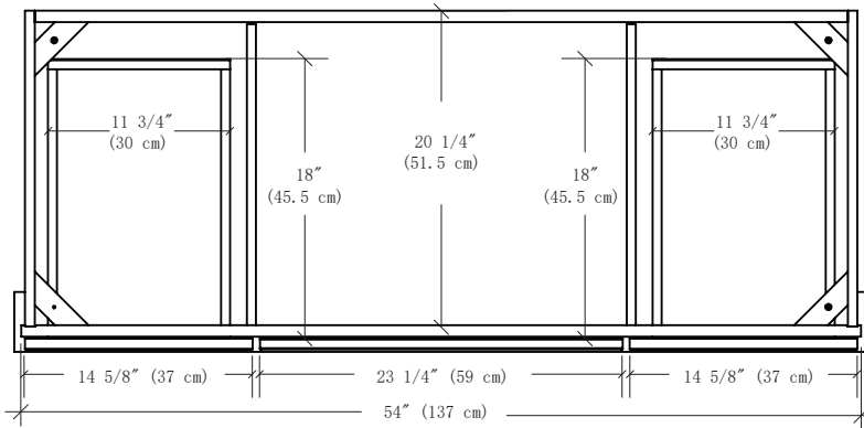
Front View / Vue avant
