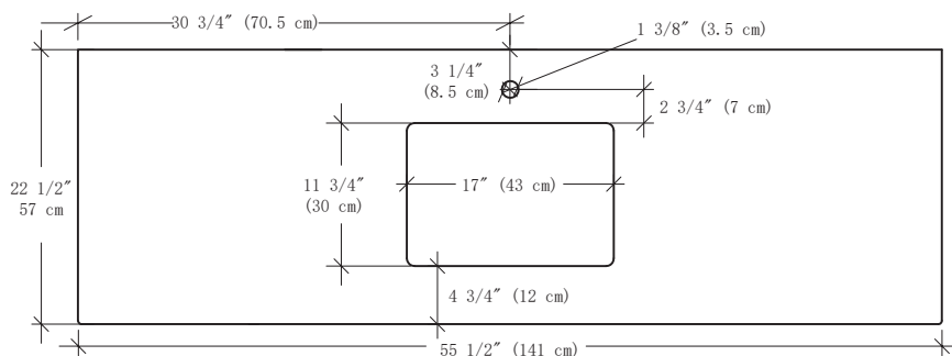
Vanity Top / Dessus du meuble-lavabo
