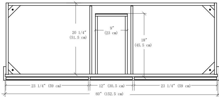
Top View / Vue de haut
